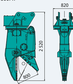
Pince de démantèlement lourd KV800PR
